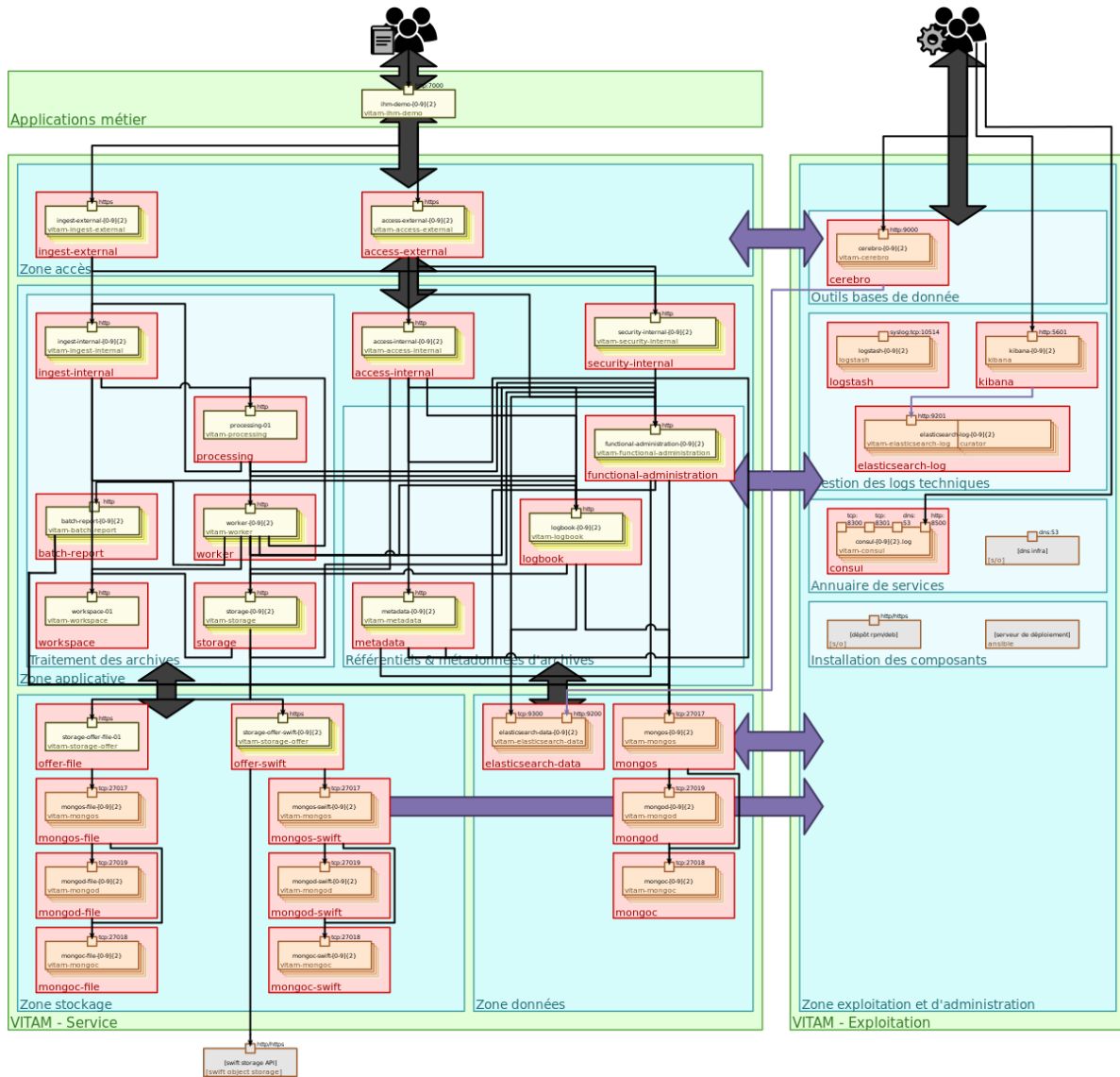
Fig. 9 – Architecture technique : délimitation par zones
